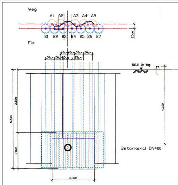
Anordnung der Bohrungen
